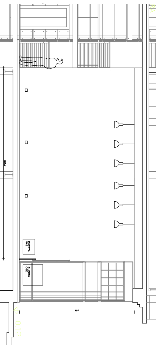
ALZADO
